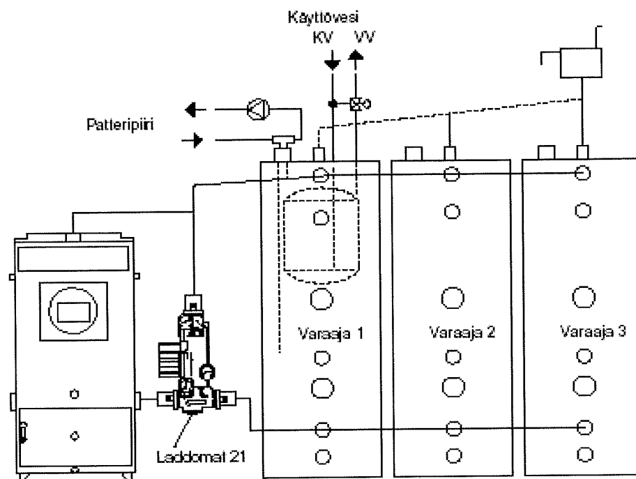
Periaatepiirros
